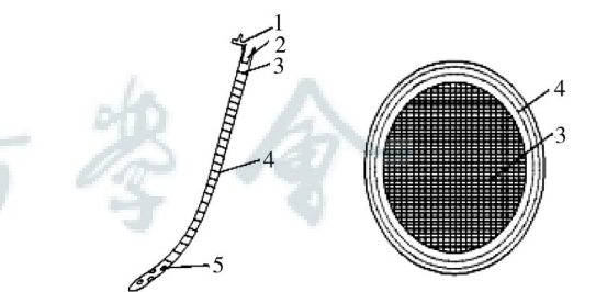
1. 环扣 2. 胃管灌注口 3. 过滤器 4. 胃管主体 5. 侧孔 图1 具有过滤功能的胃管及过滤网示意图
